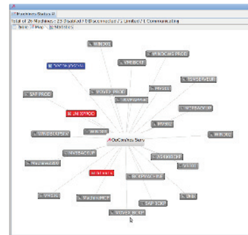
Architecture centralisée
